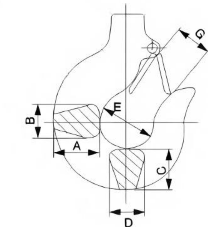
Hook 吊钩
